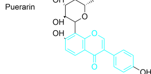
Puerarin
