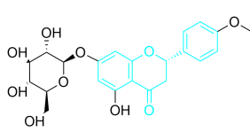
Tilianin
