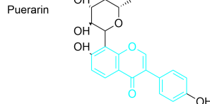
Puerarin
