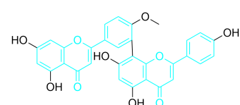
ginkgetin
