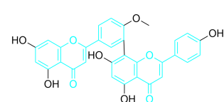
ginkgetin
