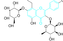
Icariin
