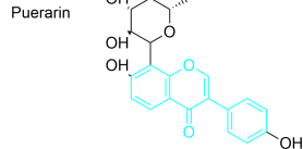
Puerarin
