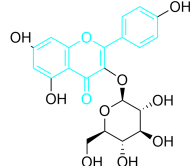
Tilianin
